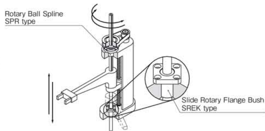
5. ábra Fügőleges robot kar Fig. 5. Vertical robot arm Fig. 5. Brat robotizat vertical
