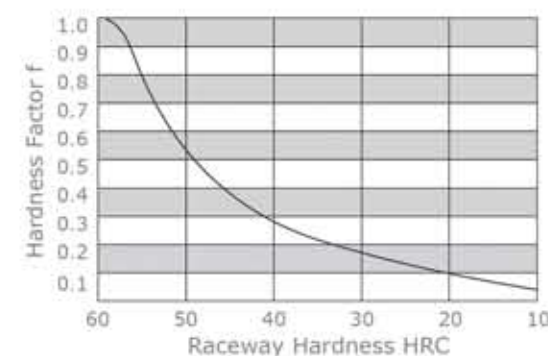
1. ábra Keménységi tényező (fH) Fig. 1. Hardness factor (fH) Fig. 1. Factorul de duritate (fH)
